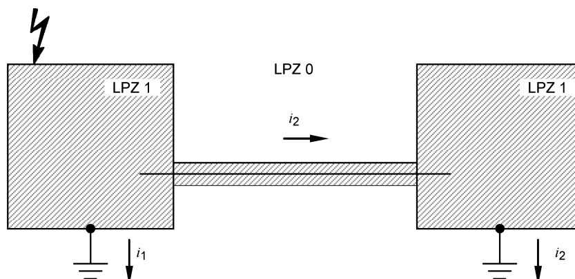
Bild 1 – Beispiel für die Verbindung von Blitzschutzpotentialausgleichszonen mit geschirmten Kabeln oder geschirmten Kabelkanälen
